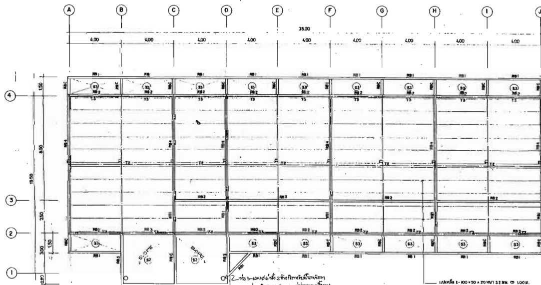
แปลนโครงสร้างชั้นกลาง ขนาดจริง
