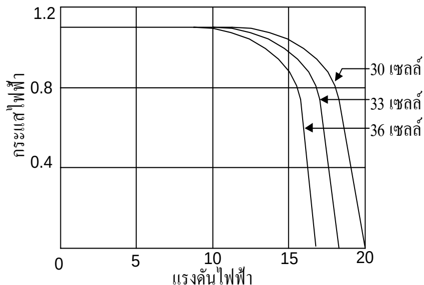
รูปที่ 5-ก ผลของจำนวนเซลล์ต่อคุณสมบัติทางไฟฟ้าของเซลล์แสงอาทิตย์
