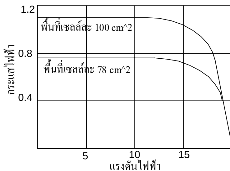
รูปที่ 6-ก ผลของพื้นที่เซลล์ต่อคุณสมบัติของเซลล์แสงอาทิตย์
